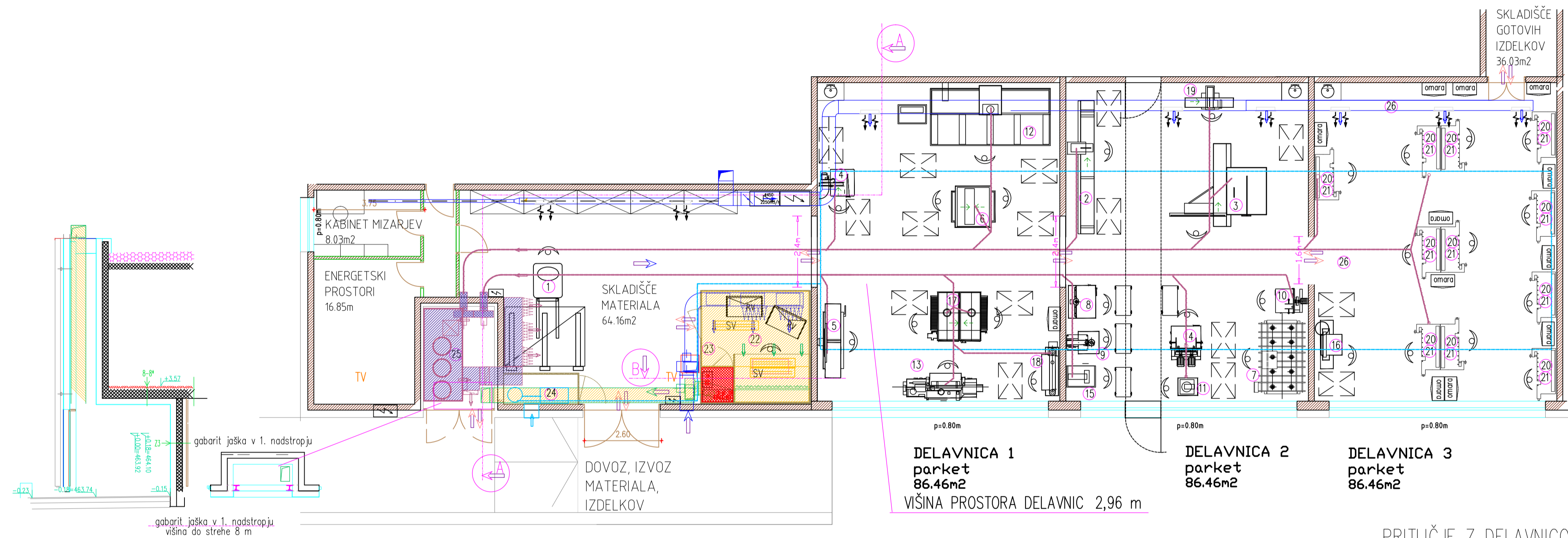
PRITLIČJE Z DELAVNICO M 1:100
